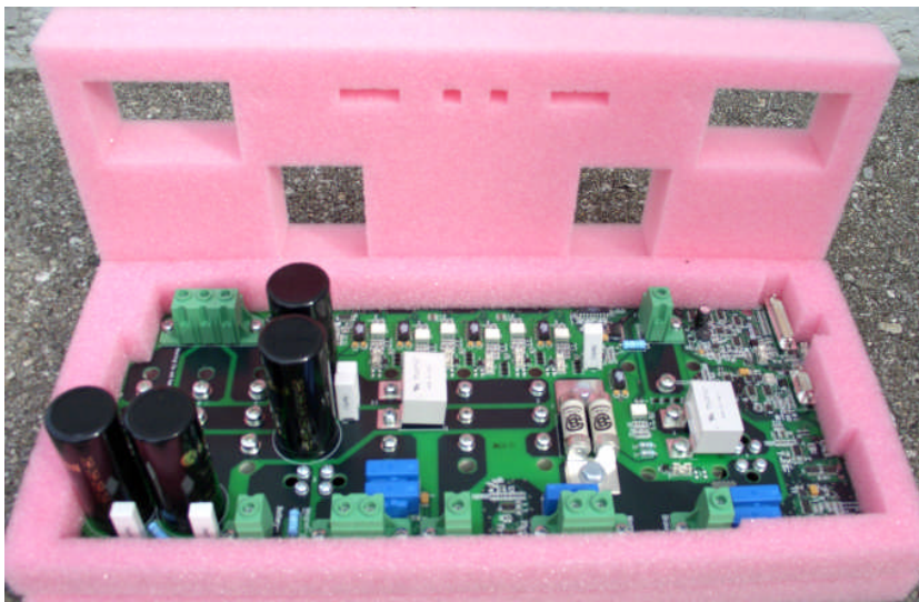
Figure 1: PowerPick Board in der schützenden Schaumstoffverpackung
